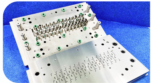
Blanking die
