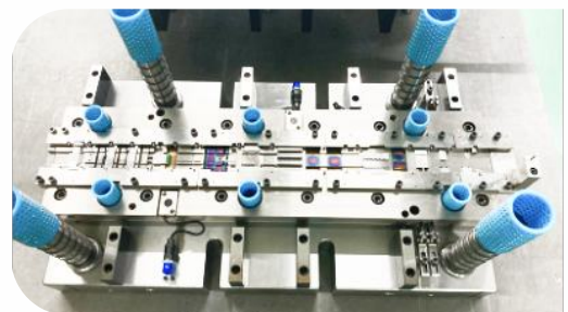
Progressive die
